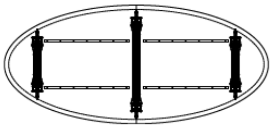
Forme d'ellipse
